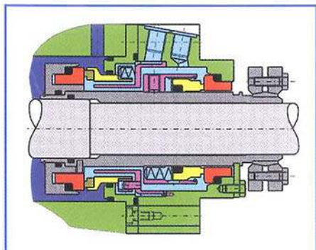
Idejni nacrt
